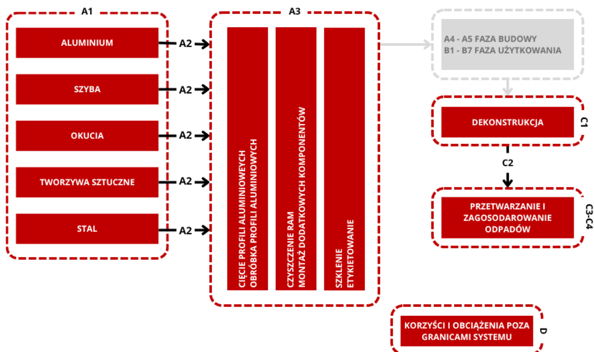
Rysunek 5.1: Granice systemu dla charakterystyki środowiskowej przeciwpożarowych ścian osłonowych
